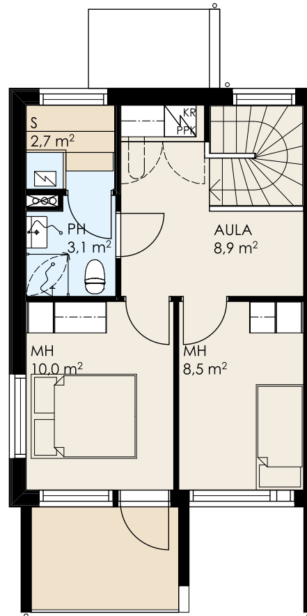
2. KERROS
