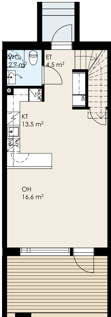
1. KERROS
